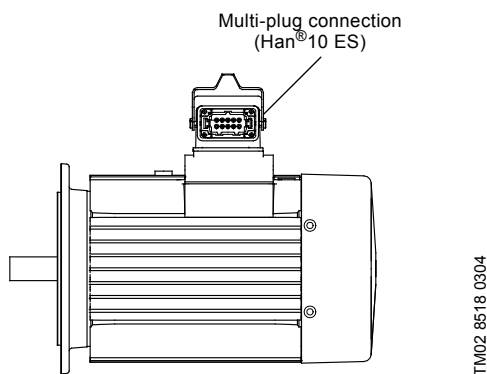
Fig. 33 Multi-plug type Han® 10 ES
